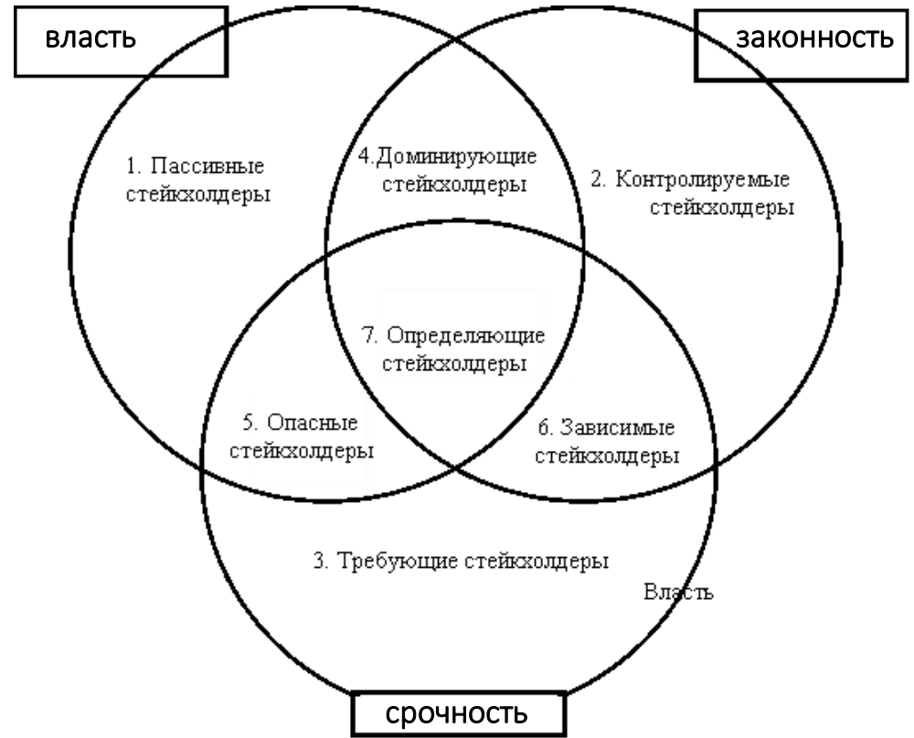
Модель Митчелла-Агле-Вуда
